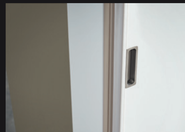
Detail: Ultraflacher Zargenfalz mit Magnetfallschließblech
